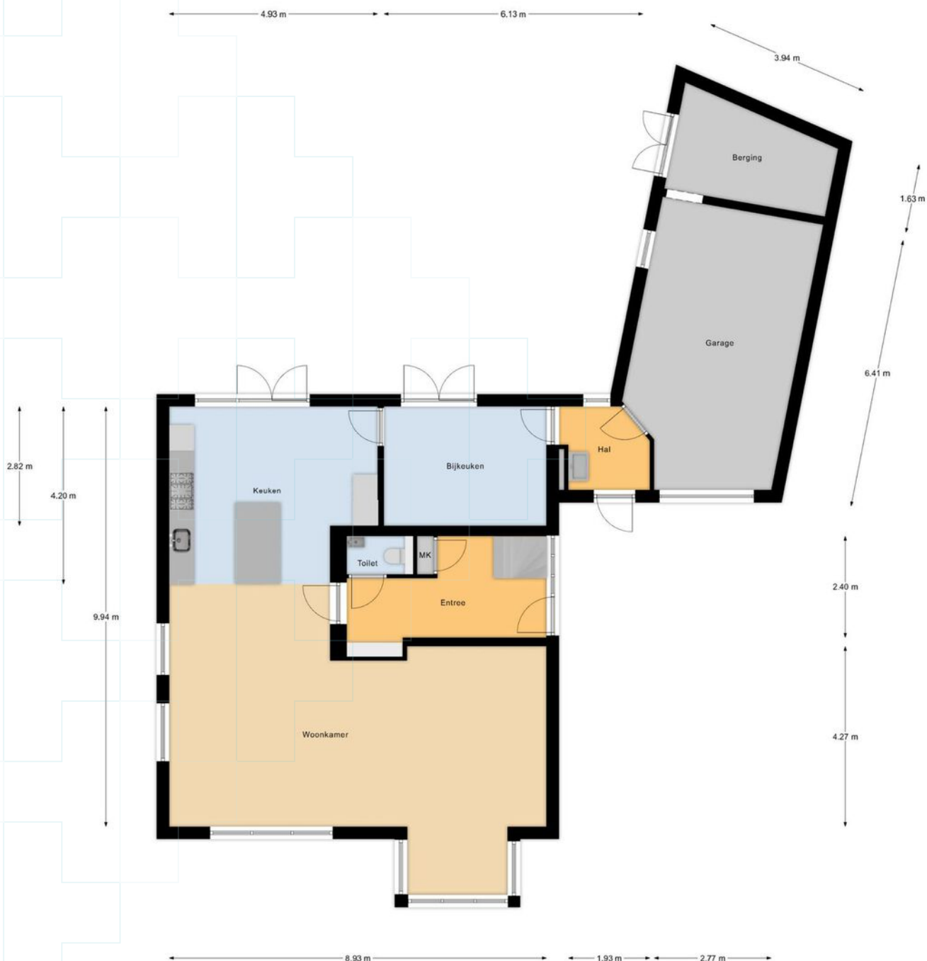
Begane Grond
