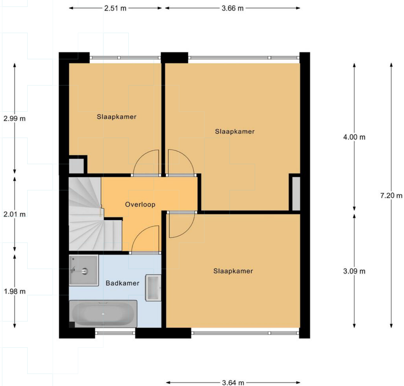
1e Verdieping
