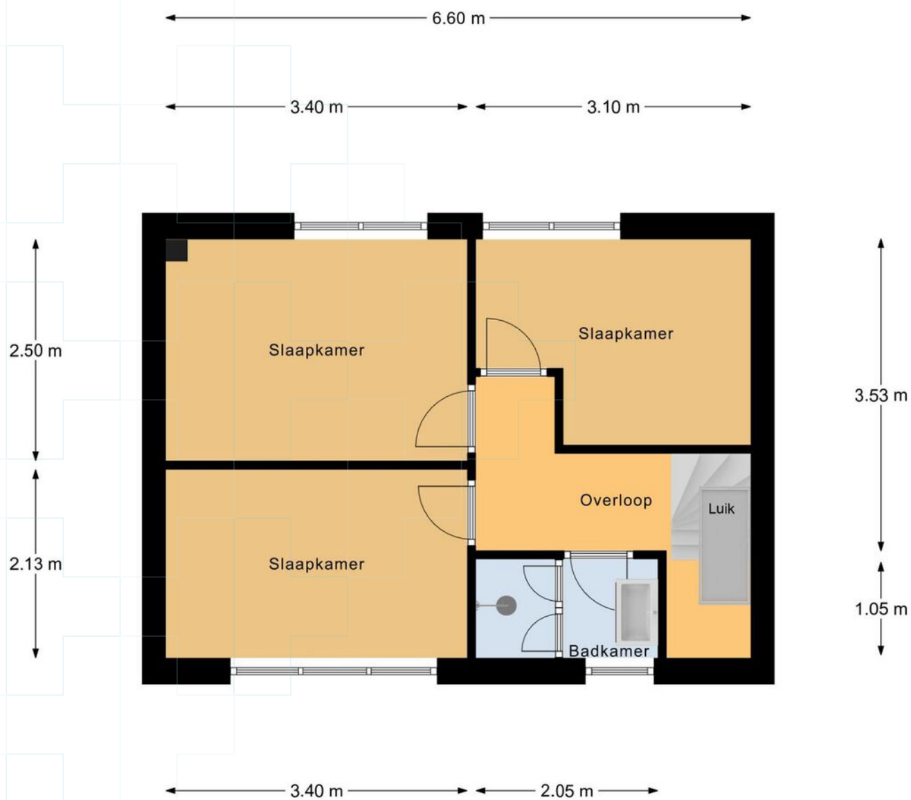
1e Verdieping
