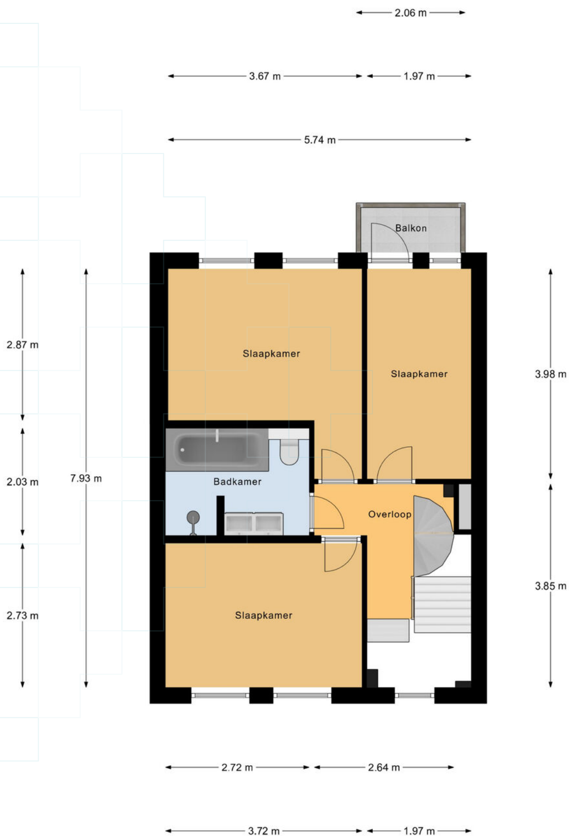
1e Verdieping
