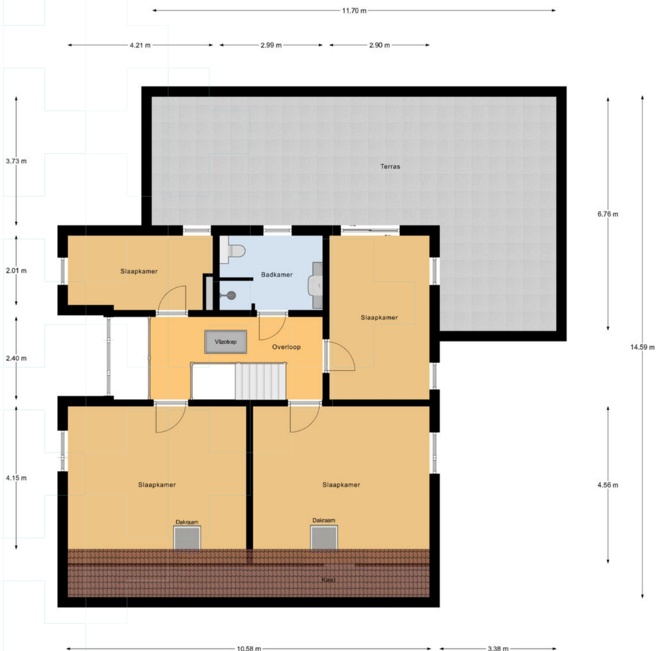
1e Verdieping
